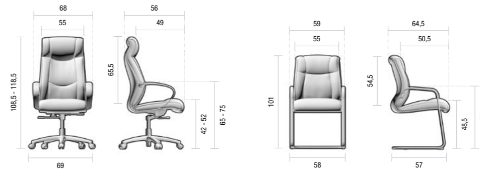
Silla de dirección Cadira de direcció / Siège direction / Executive chair / Chfessessel Stuhl.
